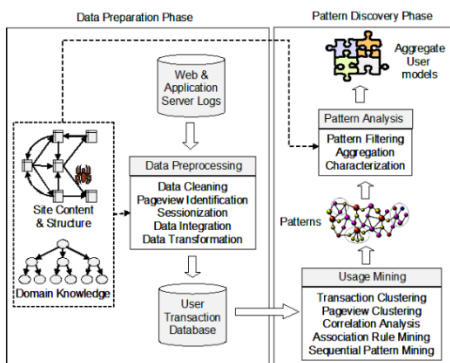
Fig. 2. Tahapan proses pada web usage mining (bing liu.2011.web data mining.second edition.springer.page 528)[11]
