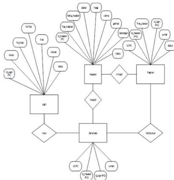
Gambar 9 : ERD Aplikasi Pemesanan Menu pada Smart Café
